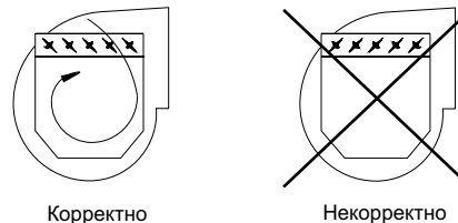
Рисунок 7. Ориентировка лопастей демпфера по отношению к направлению вращения вентилятора
