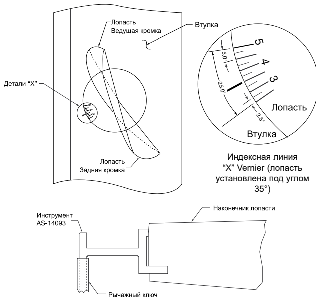
Рис. 10. Регулировка угла лопасти VJ
