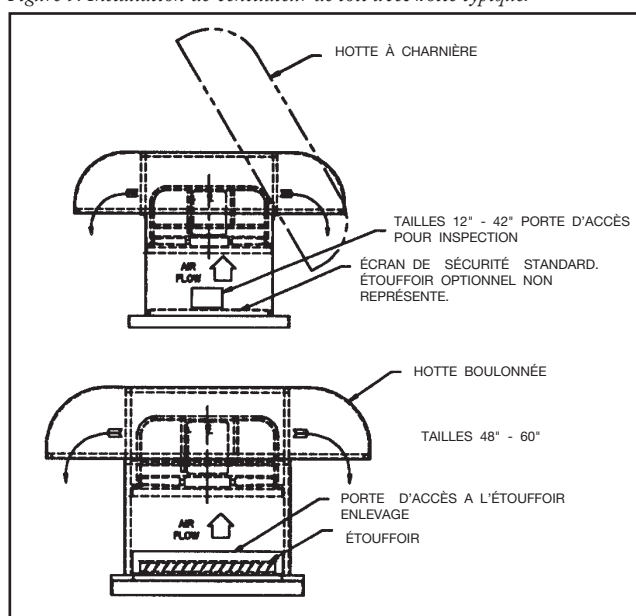
Figure 9. Installation de ventilateur de toit avec hotte typique.
