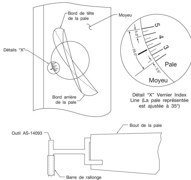
Figure 10. Alignement de l'angle des pales pour le type VJ
