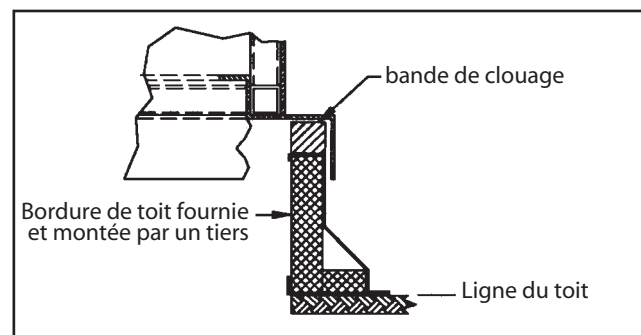
Figure 8. Montage du ventilateur de toit sur le capuchon de bordure
