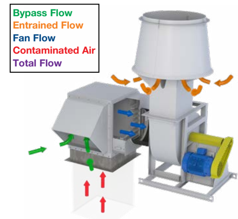
LAB EXHAUST FAN
