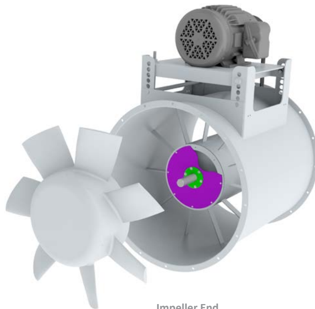
Impeller End
